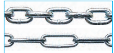
Schweiß - und Gliederketten nach DIN 5685, DIN 766 und DIN 763 Welded link chains according to DIN 5685, DIN 766 and DIN 763
