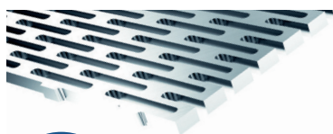
Langlochung gestanzt z.B. 1,4 mm Schlitzweite in Edelstahl der Stärke 3 mm
